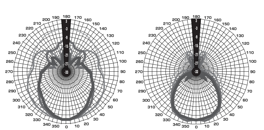
HORIZONTAL POLAR DIAGRAM — 250 — 500 — 1000 — 2000 — 4000 — 8000 — 12500 — 16000
